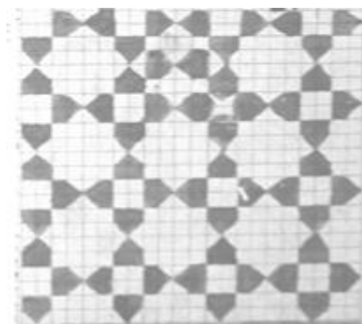
تصویر ۳. تصویری از ترسیم گره هشت چلیپا در شبکه شطرنجی در طومار میزرا علی اکبر در کتاب هندسه و تزیین در معماری اسلامی (نجیب‌اوغلو، ۱۳۸۸)
